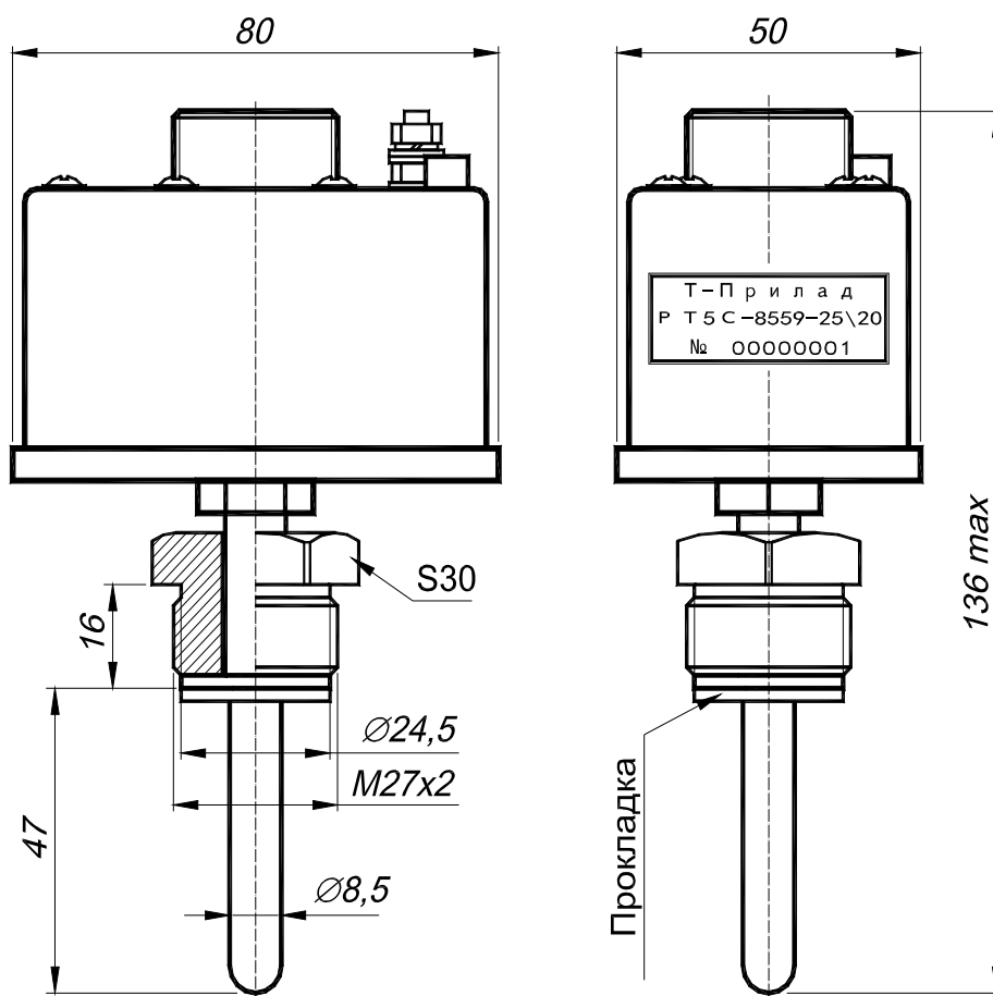
Малюнок 1 – Габаритні розміри РТ5С-8559.
