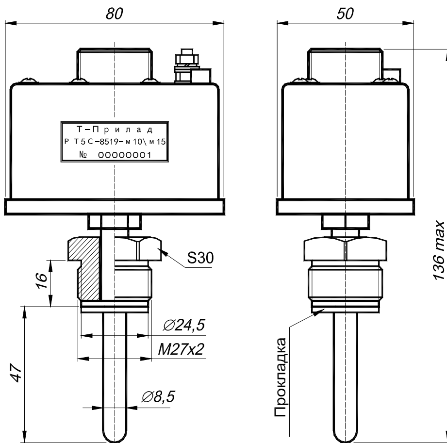
Малюнок 1 – Габаритні розміри РТ5С-8519.
