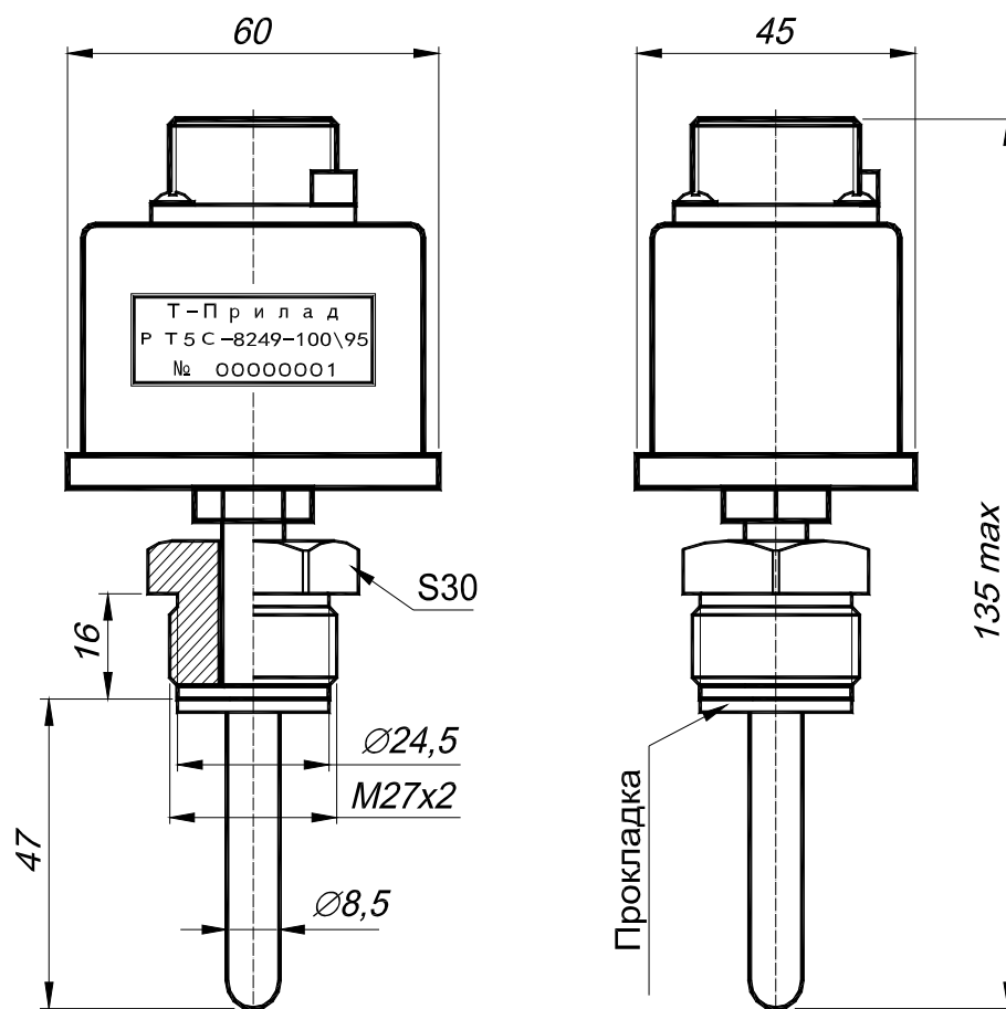
Малюнок 1 – Габаритні розміри РТ5С-8249.
