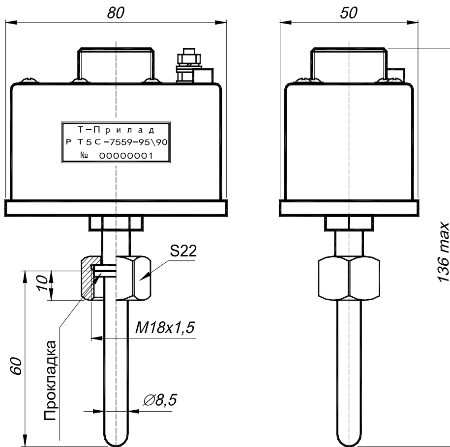
Рисунок 1 – Габаритные размеры PT5C-7559.
