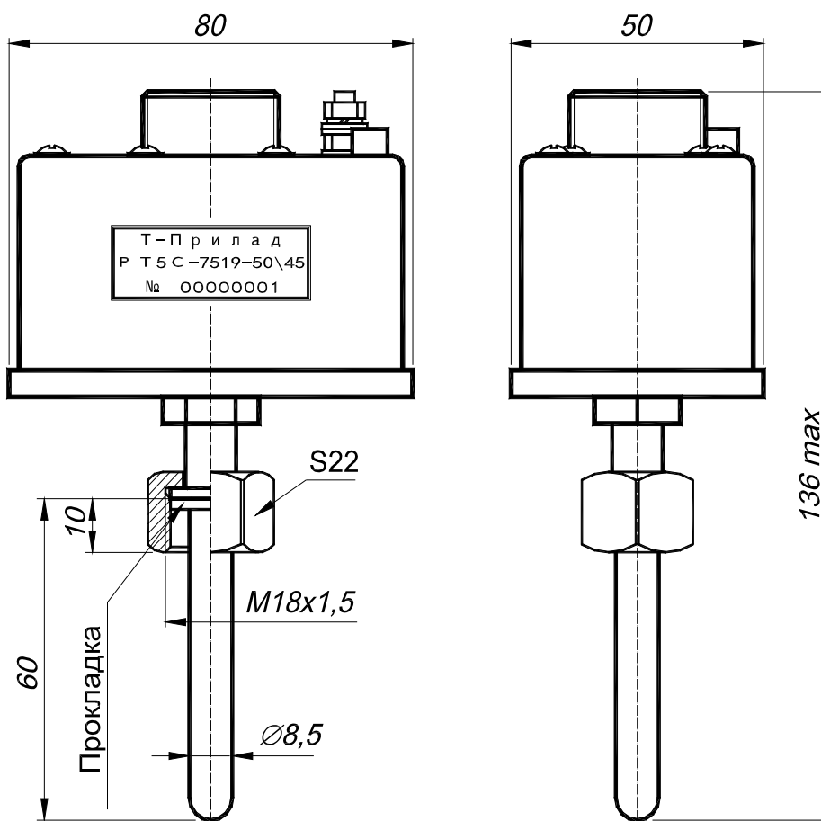
Малюнок 1 – Габаритні розміри РТ5С-7519.
