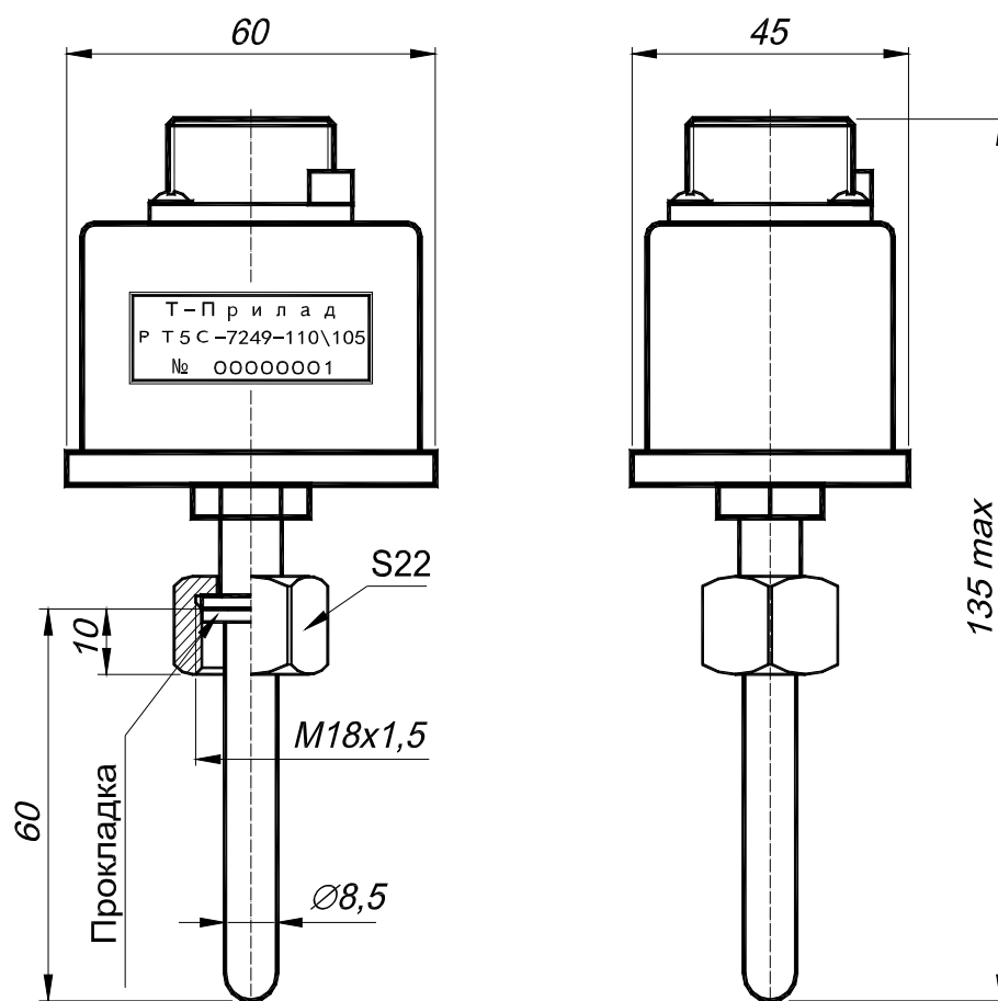
Малюнок 1 – Габаритні розміри РТ5С-7249.
