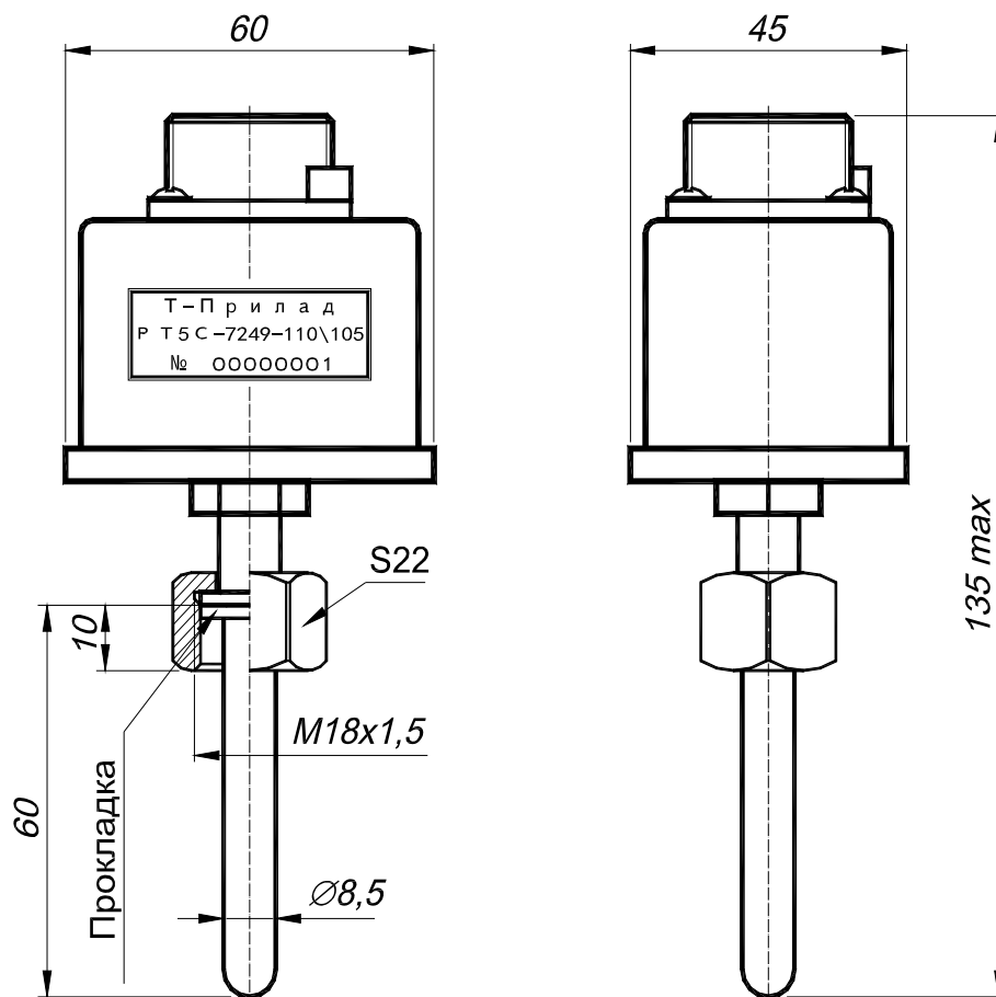
Рисунок 1 – Габаритные размеры PT5C-7249.
