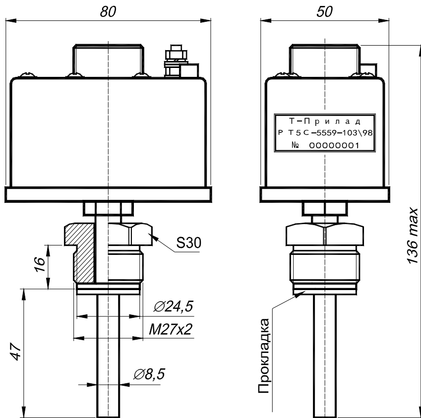
Малюнок 1 – Габаритні розміри РТ5С-5559.
