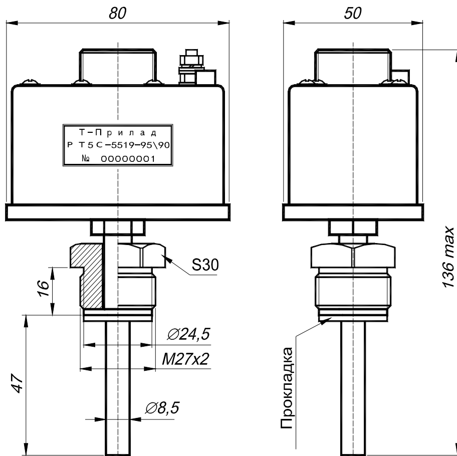
Малюнок 1 – Габаритні розміри РТ5С-5519.
