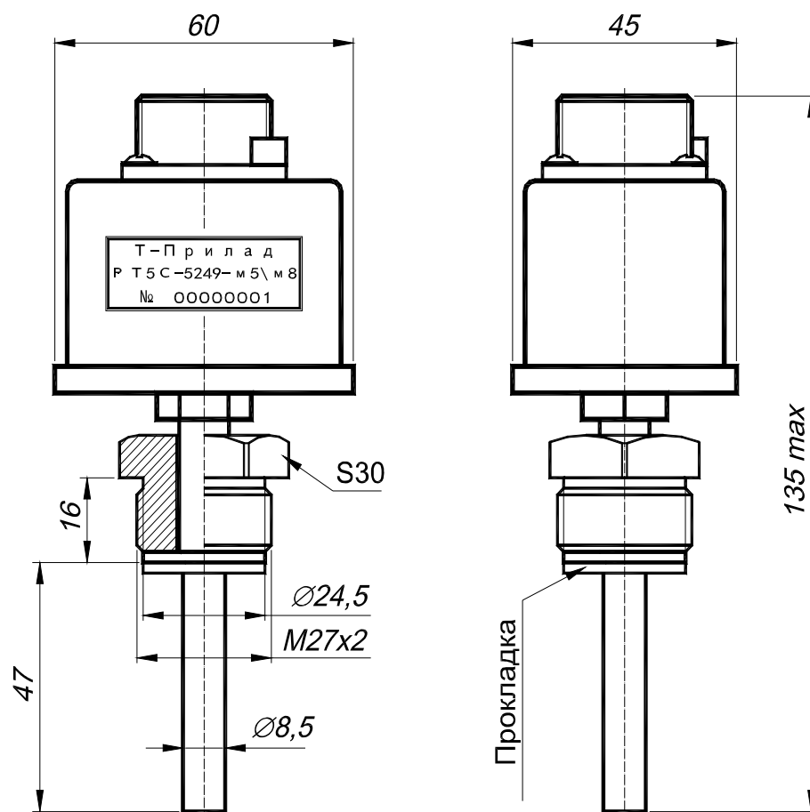
Рисунок 1 – Габаритные размеры РТ5С-5249.
