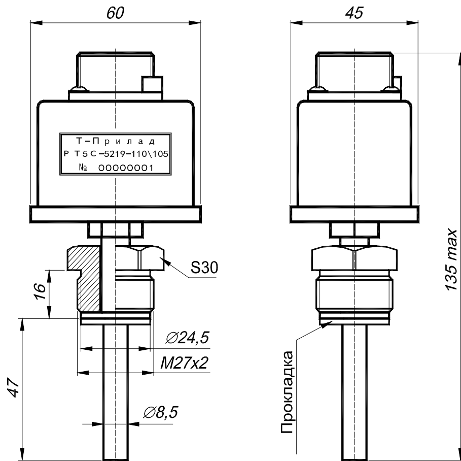
Малюнок 1 – Габаритні розміри РТ5С-5219.
