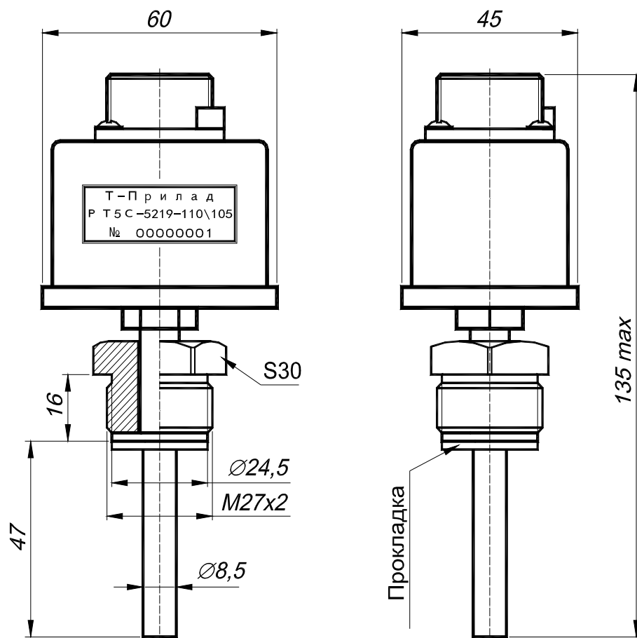
Рисунок 1 – Габаритные размеры РТ5С-5219.
