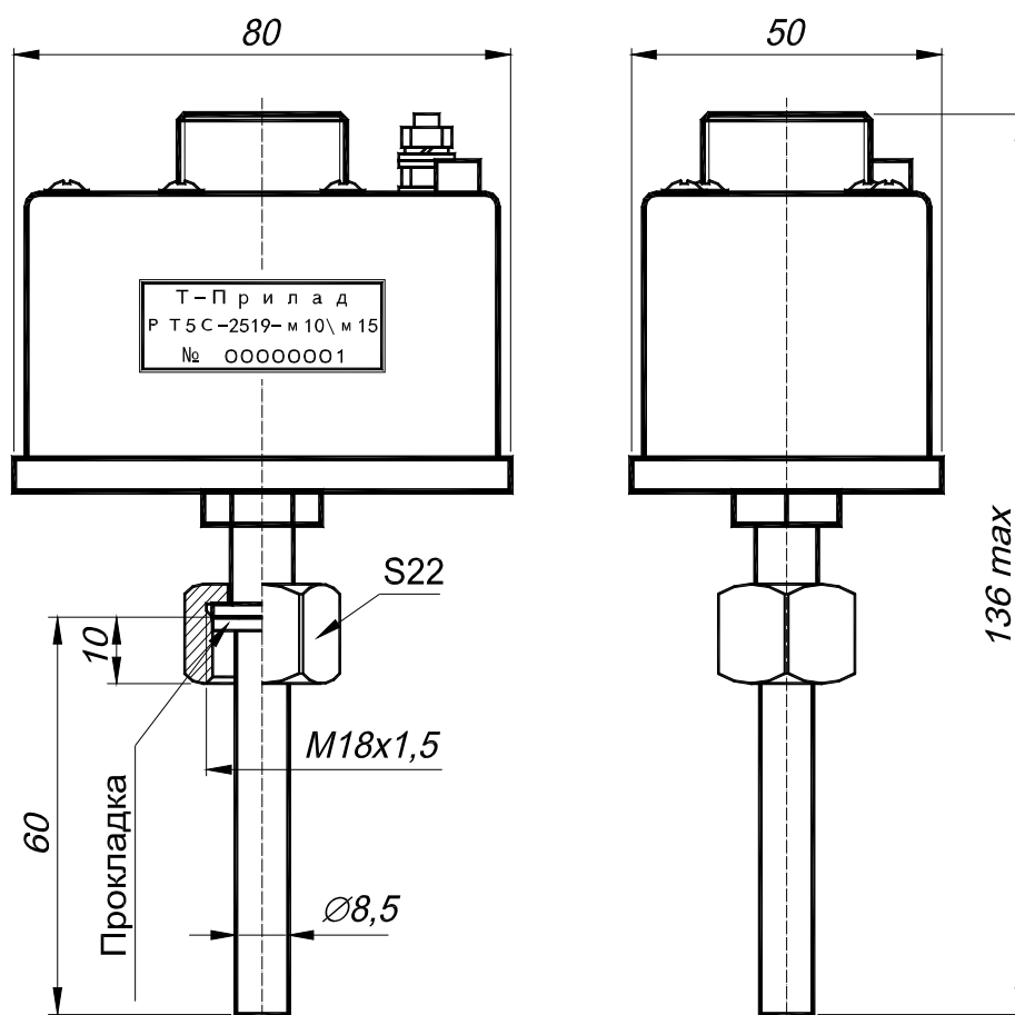
Малюнок 1 – Габаритні розміри РТ5С-2519.
