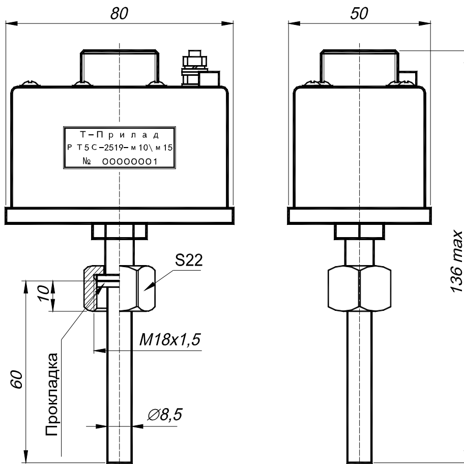
Рисунок 1 – Габаритные размеры PT5C-2519.
