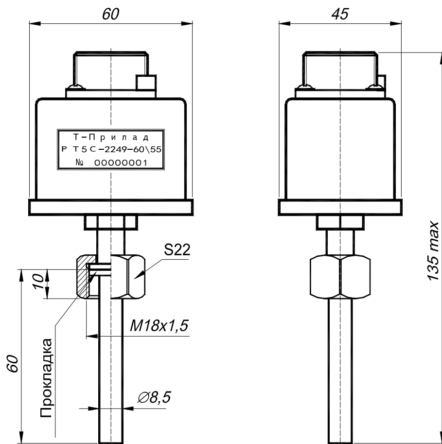
Рисунок 1 – Габаритные размеры РТ5С-2249.
