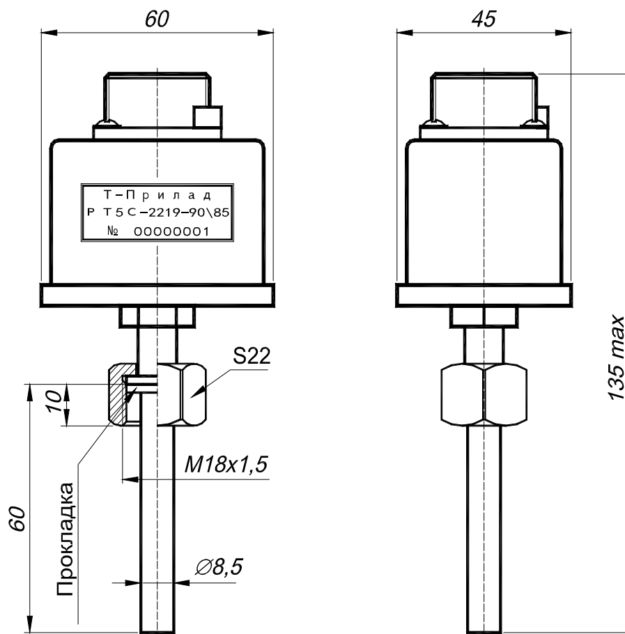
Малюнок 1 – Габаритні розміри РТ5С-2219.
