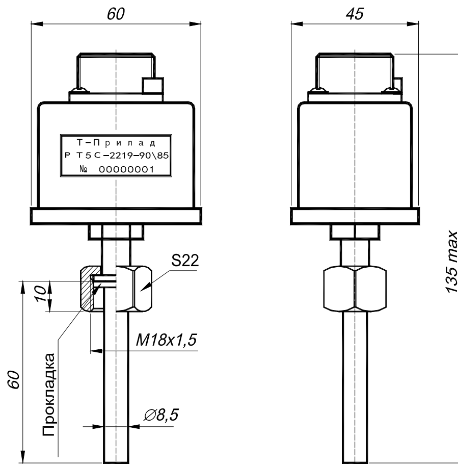
Рисунок 1 – Габаритные размеры РТ5С-2219.
