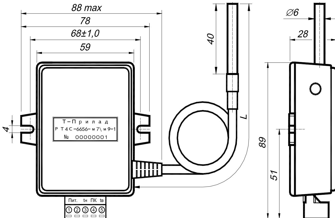
Рисунок 1 – Габаритные размеры РТ4С-6656.
