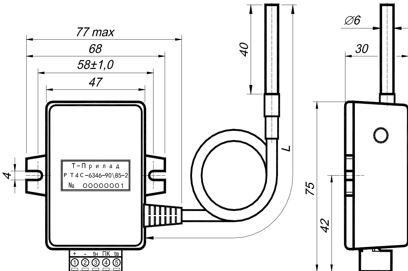
Малюнок 1 – Габаритні розміри РТ4С-6346.
