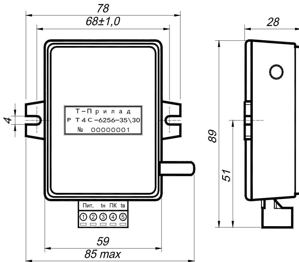
Рисунок 1 – Габаритные размеры РТ4С-6256.
