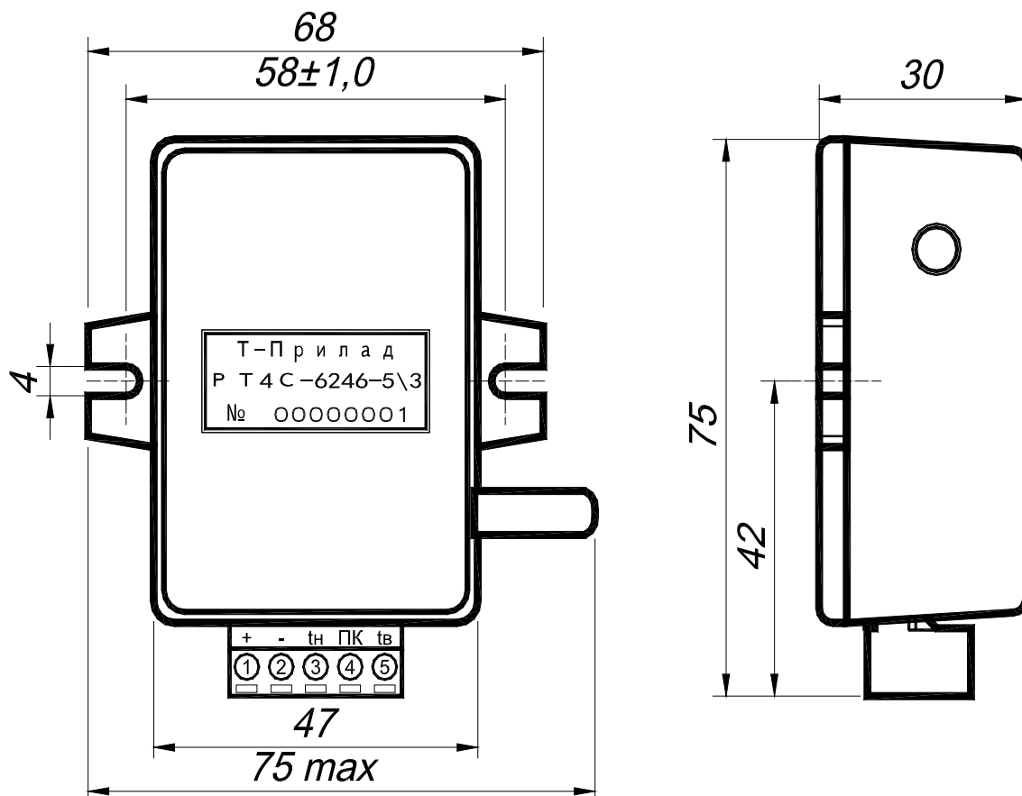
Рисунок 1 – Габаритные размеры РТ4С-6246.
