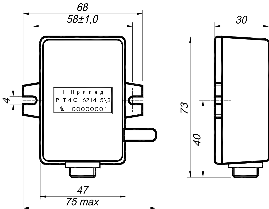
Малюнок 1 – Габаритні розміри РТ4С-6214.
