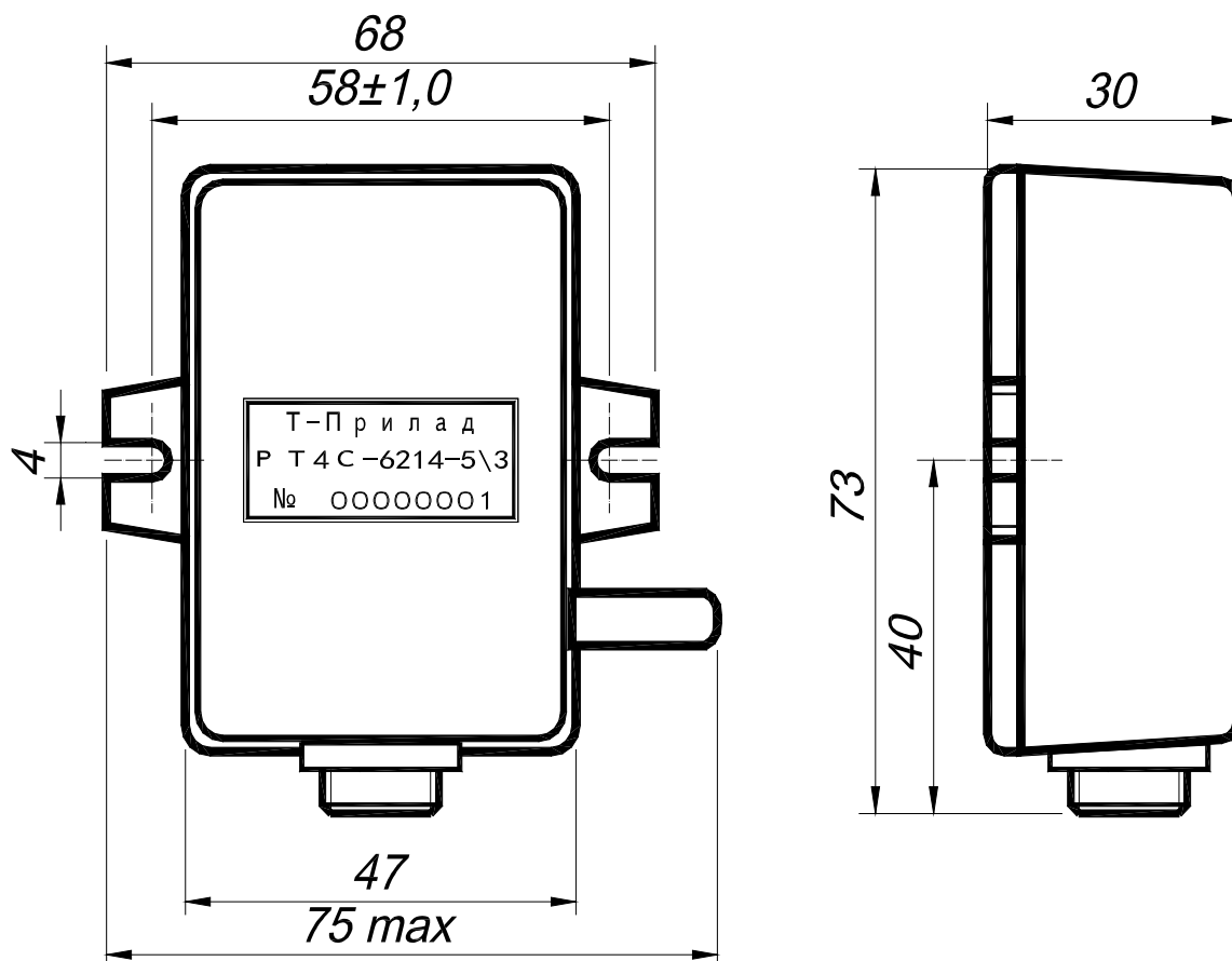
Рисунок 1 – Габаритные размеры РТ4С-6214.
