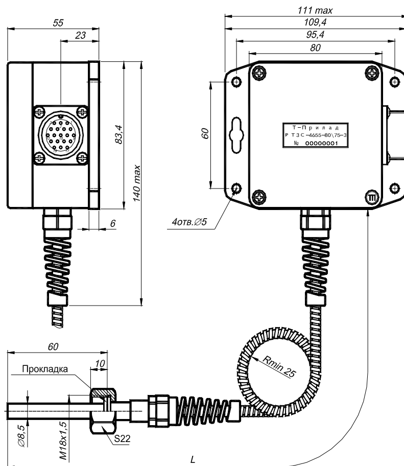
Малюнок 1 – Габаритні розміри РТЗС-4655.
