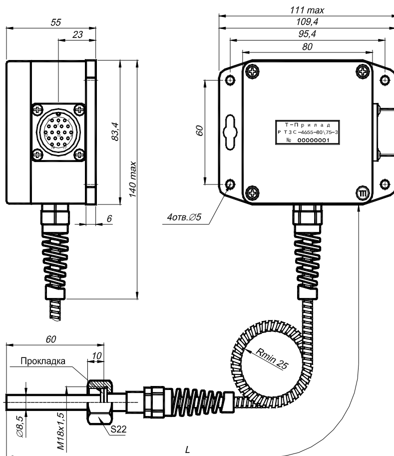
Рисунок 1 – Габаритные размеры РТЗС-4655.
