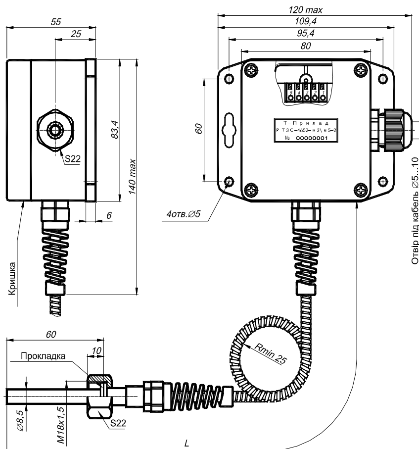
Малюнок 1 – Габаритні розміри РТЗС-4652.
