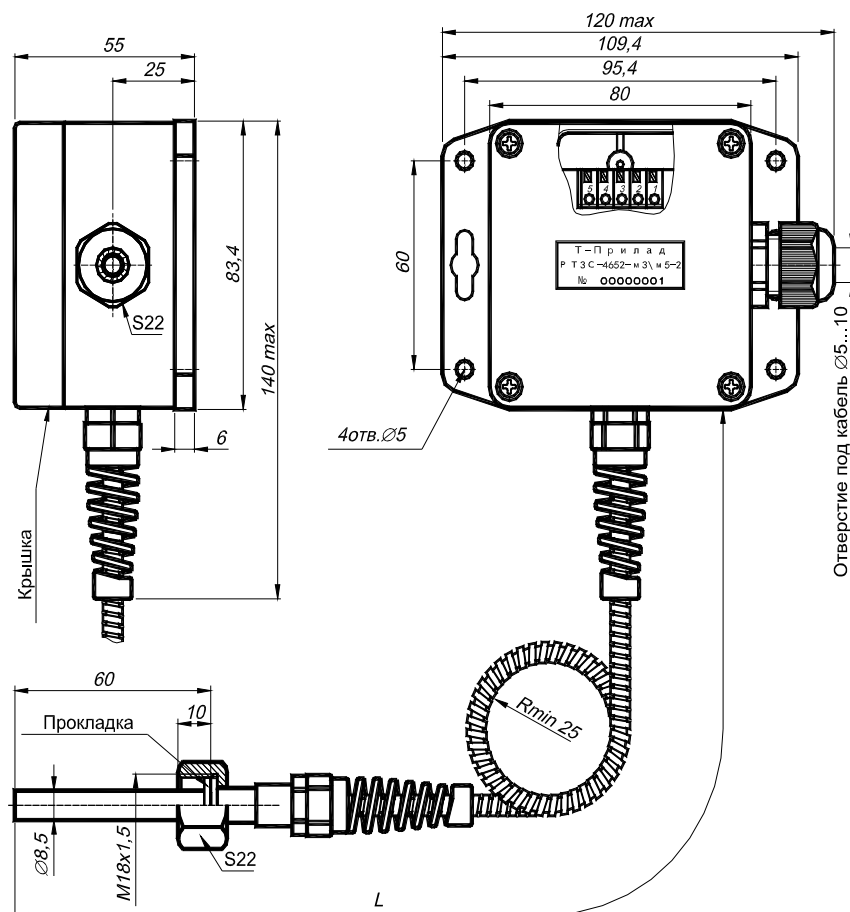
Рисунок 1 – Габаритные размеры РТЗС-4652.
