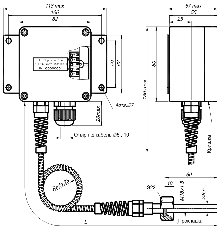
Малюнок 1 – Габаритні розміри РТЗС-4552.
