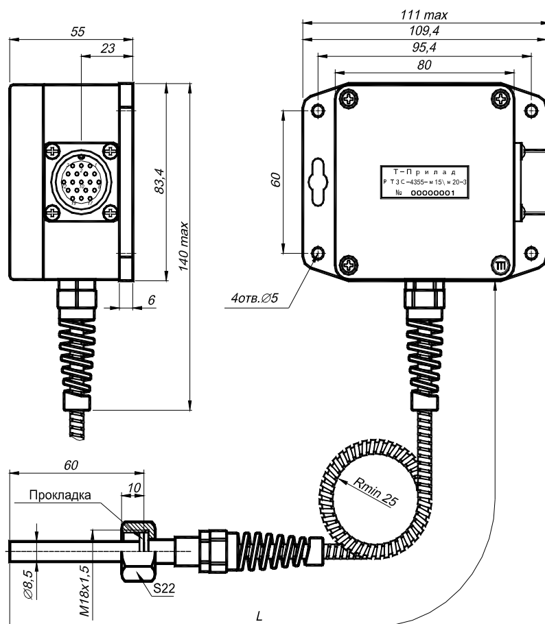
Рисунок 1 – Габаритные размеры РТЗС-4355.
