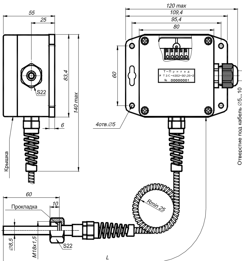
Рисунок 1 – Габаритные размеры РТЗС-4352.
