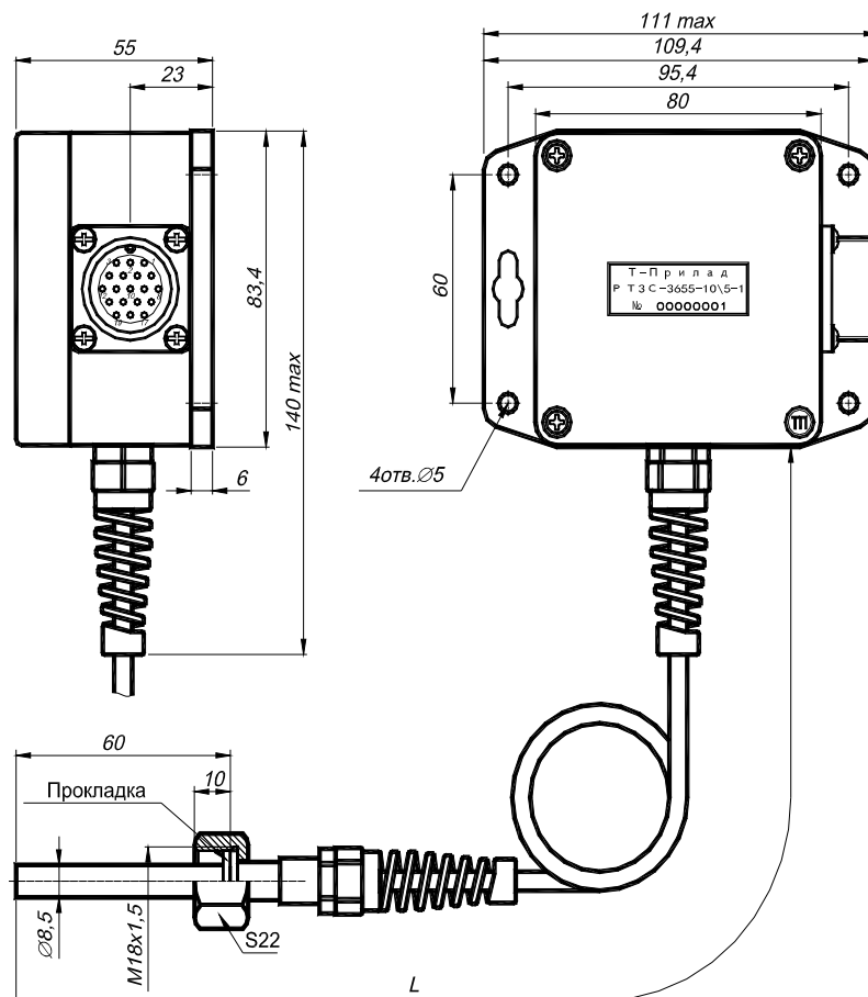
Малюнок 1 – Габаритні розміри РТЗС-3655.
