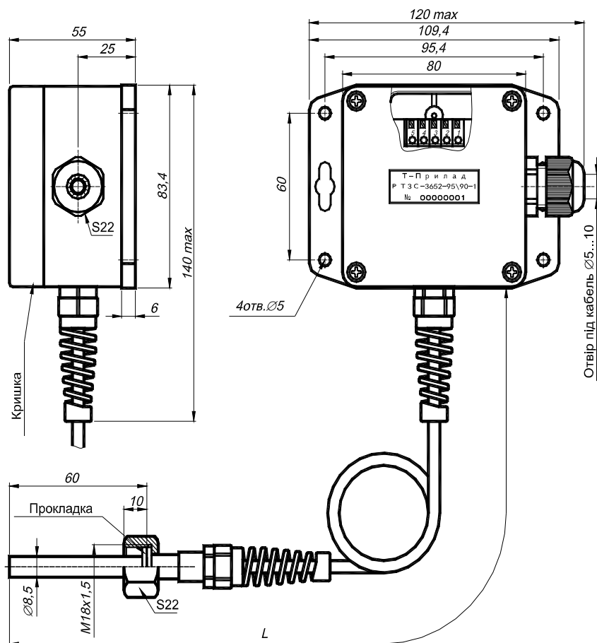
Малюнок 1 – Габаритні розміри РТЗС-3652.
