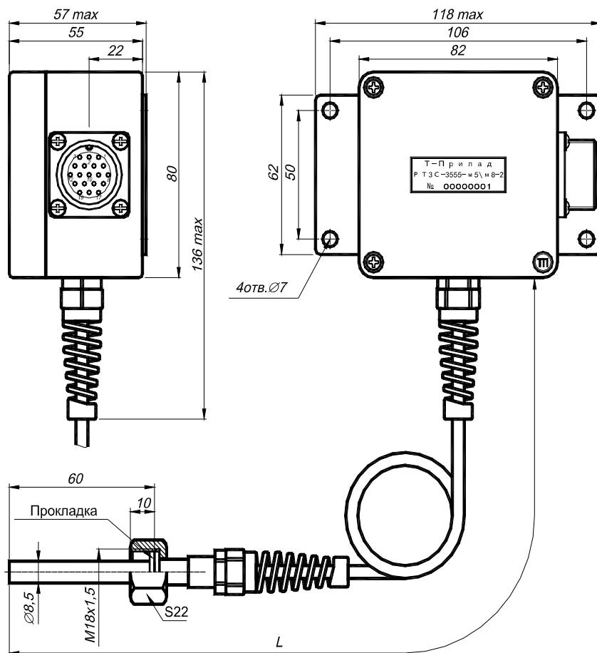
Малюнок 1 – Габаритні розміри РТЗС-3555.
