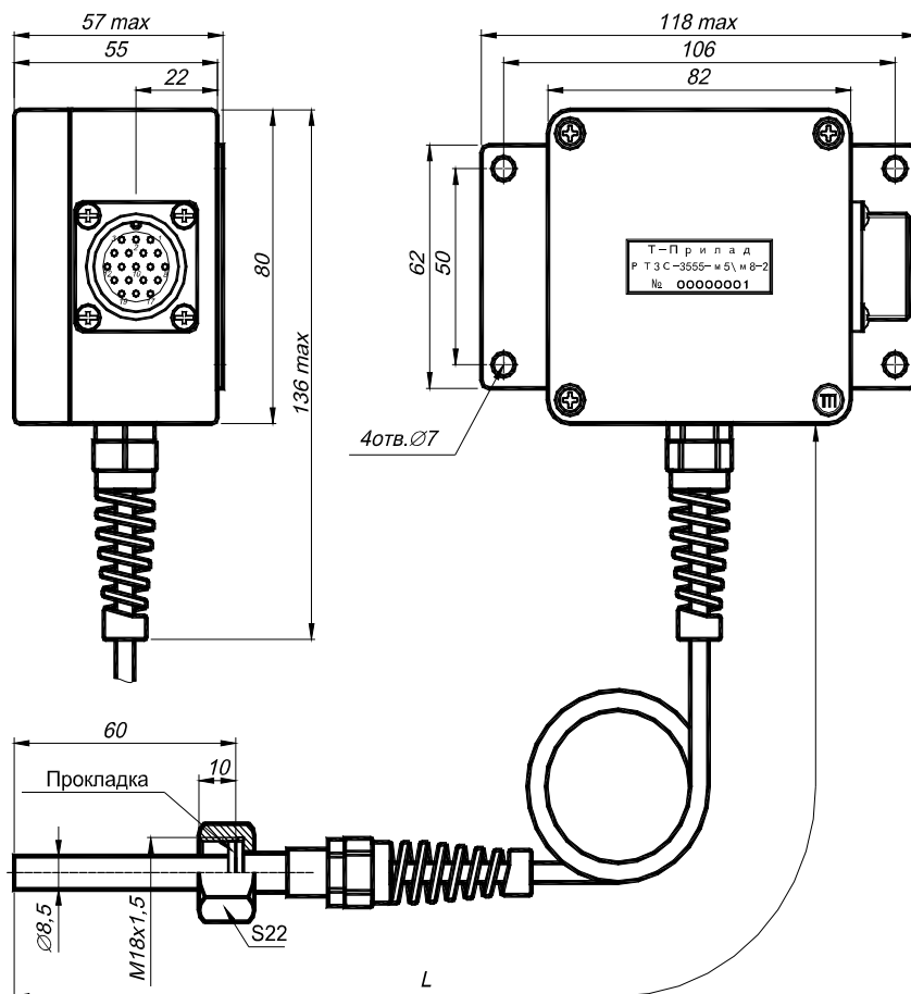
Рисунок 1 – Габаритные размеры РТ3С-3555.
