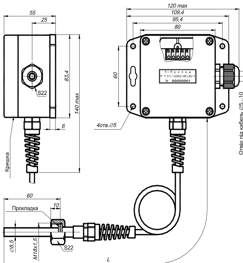
Малюнок 1 – Габаритні розміри РТЗС-3352.
