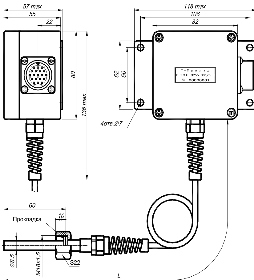
Малюнок 1 – Габаритні розміри РТЗС-3255.
