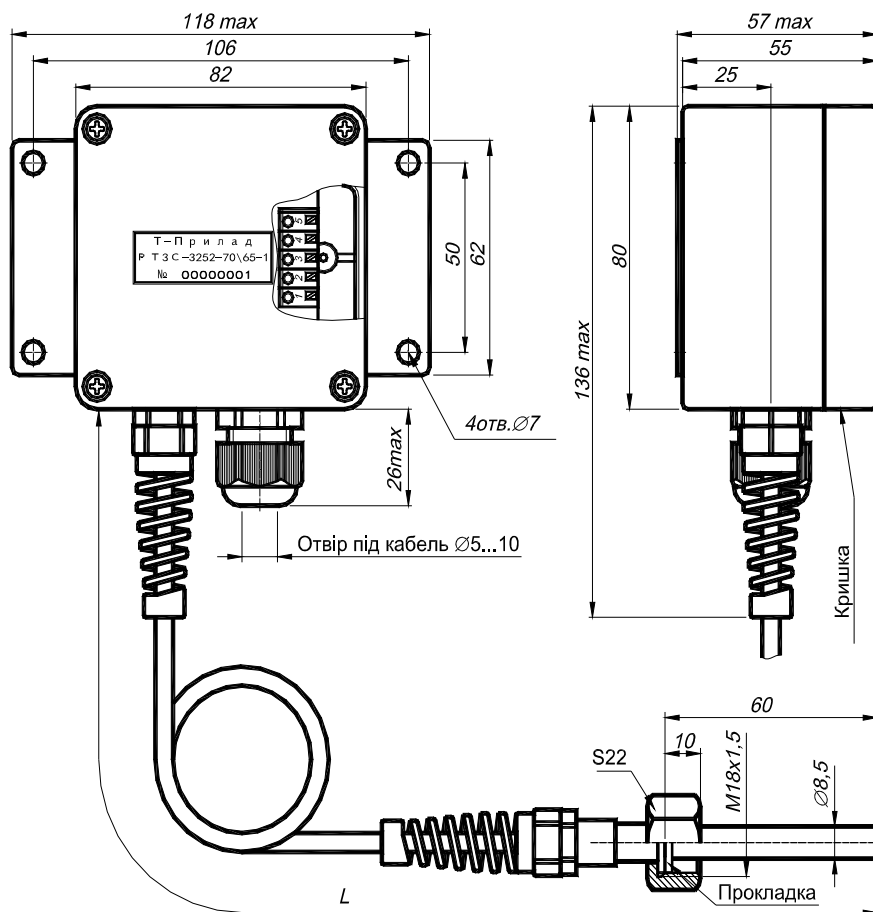
Малюнок 1 – Габаритні розміри РТЗС-3252.
