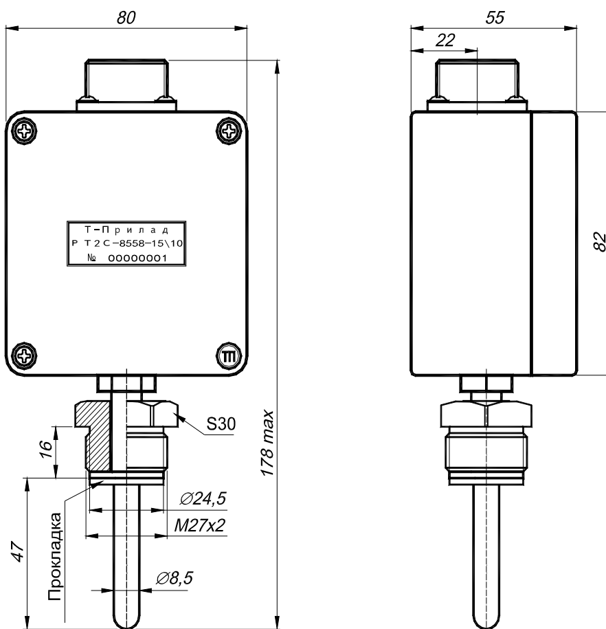
Малюнок 1 – Габаритні розміри РТ2С-8558.
