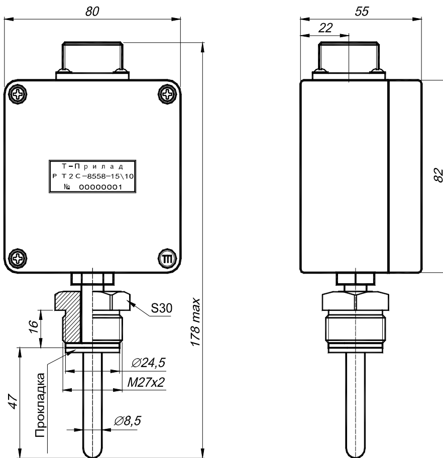
Рисунок 1 – Габаритные размеры PT2C-8558.
