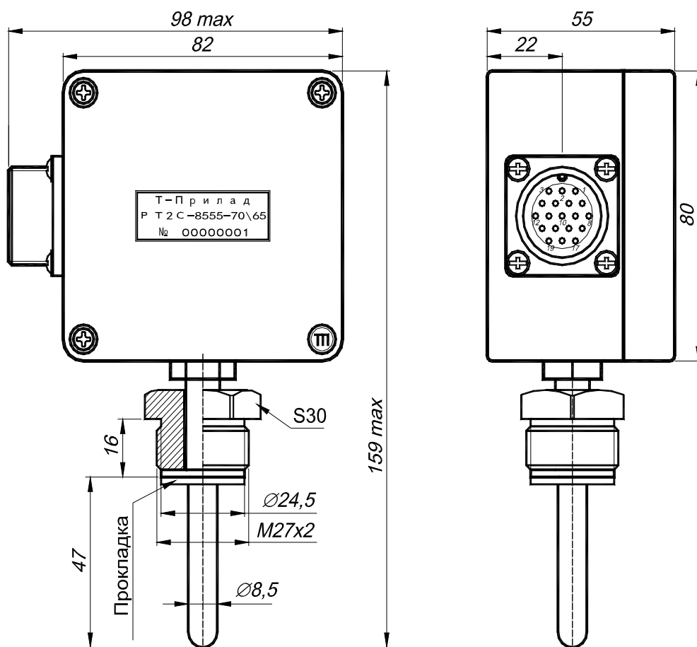
Малюнок 1 – Габаритні розміри РТ2С-8555.
