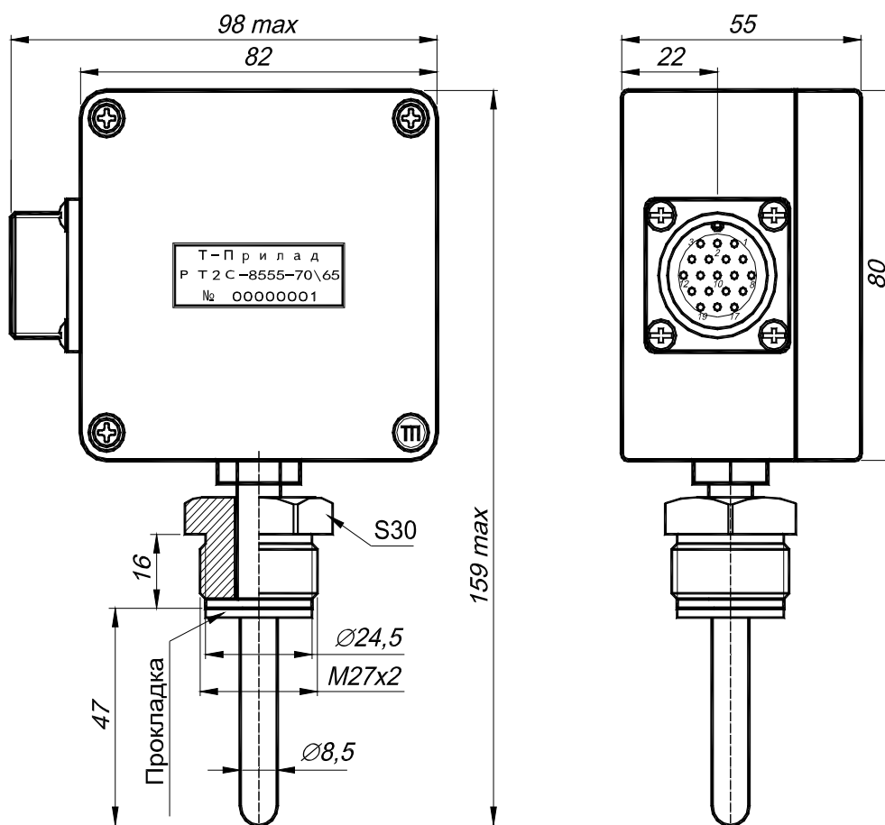
Рисунок 1 – Габаритные размеры PT2C-8555.
