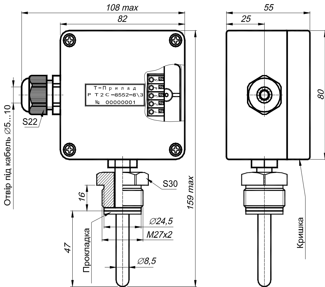
Малюнок 1 – Габаритні розміри РТ2С-8552.
