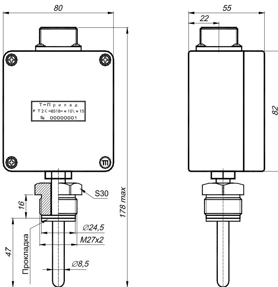
Малюнок 1 – Габаритні розміри РТ2С-8518.
