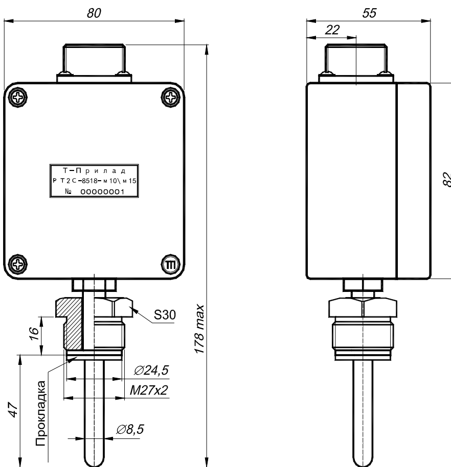
Рисунок 1 – Габаритные размеры PT2C-8518.
