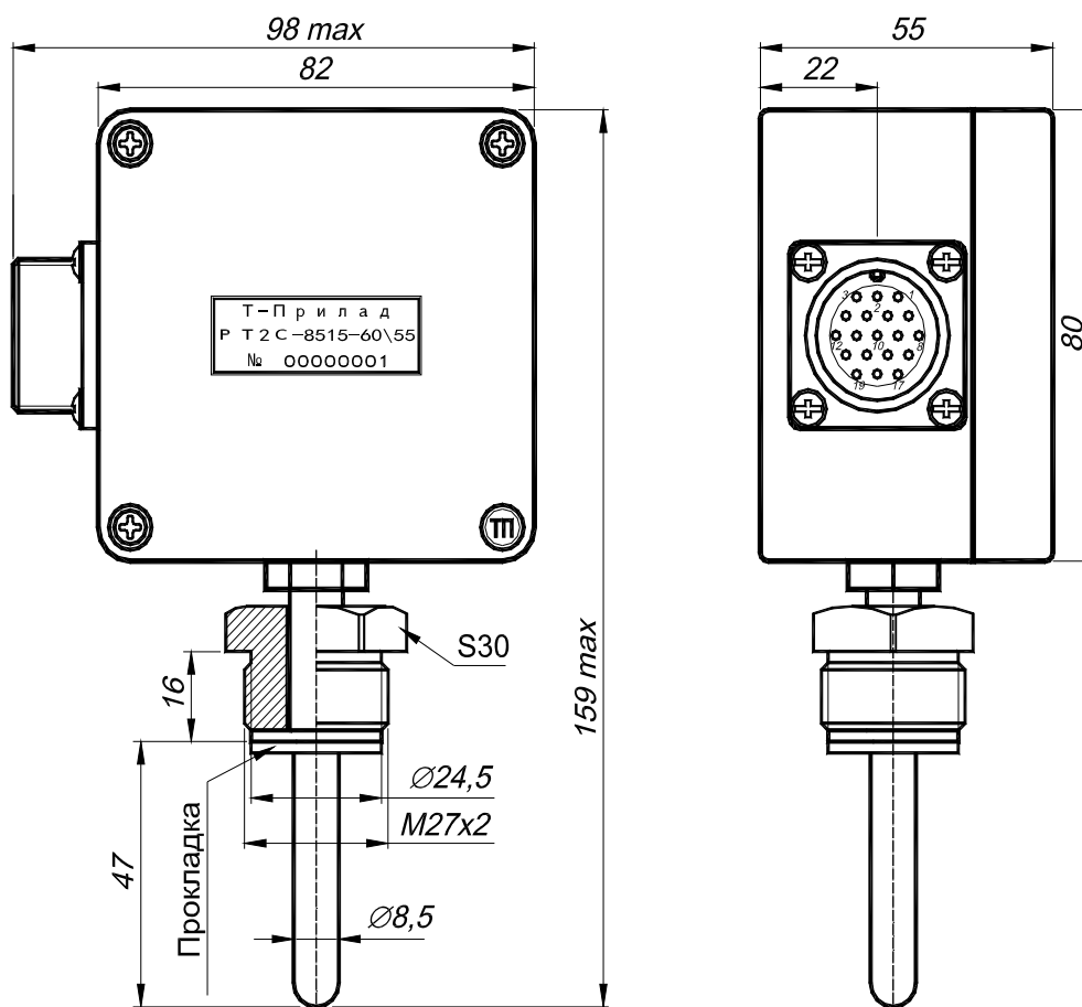
Малюнок 1 – Габаритні розміри РТ2С-8515.
