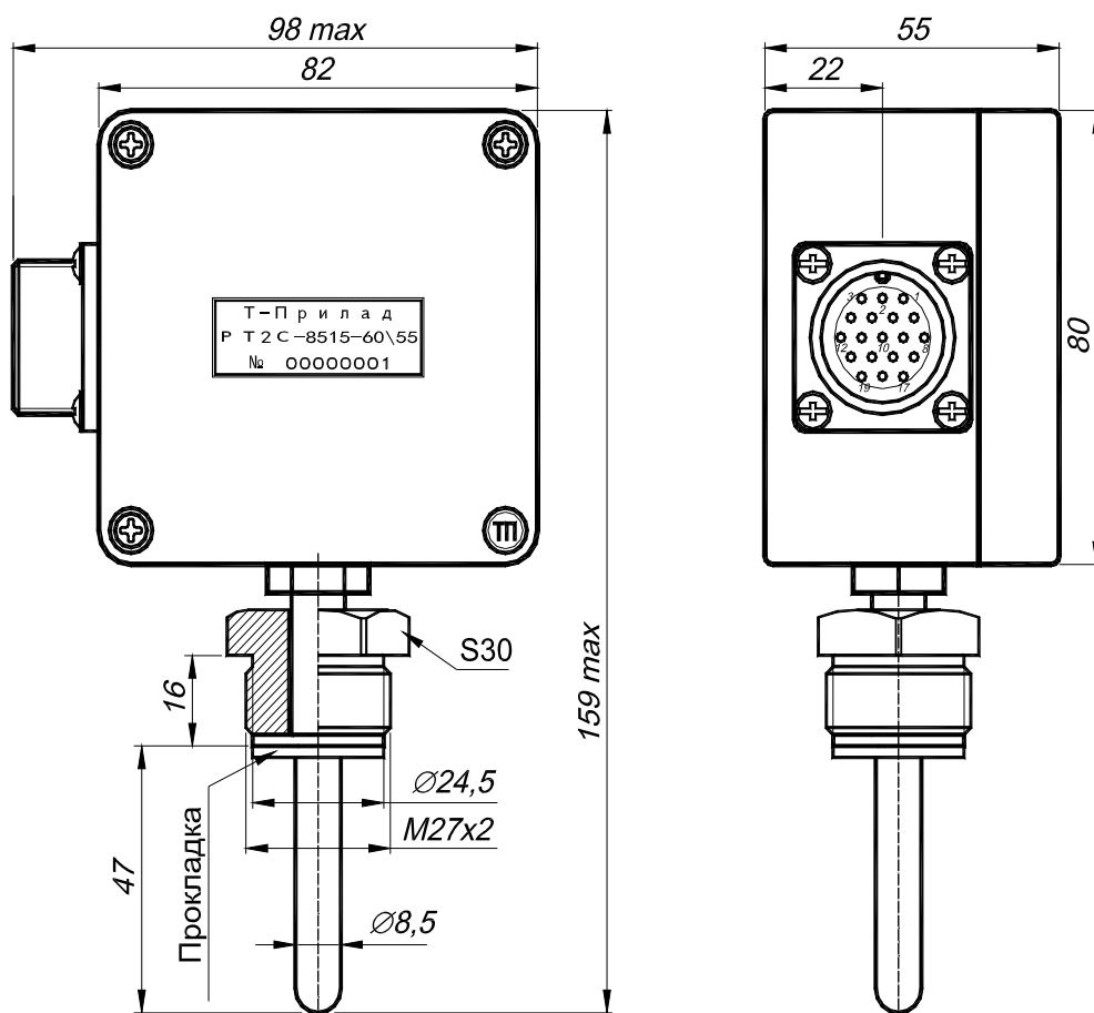
Рисунок 1 – Габаритные размеры PT2C-8515.
