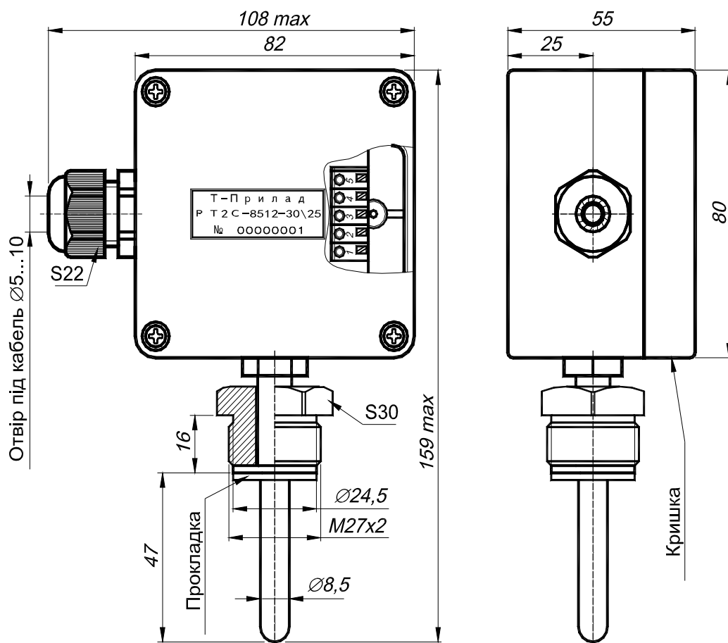
Малюнок 1 – Габаритні розміри РТ2С-8512.
