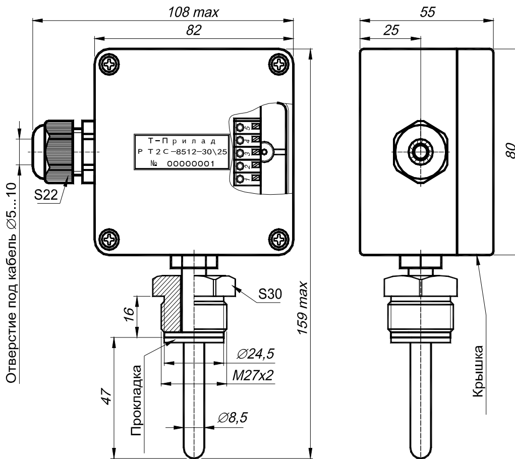
Рисунок 1 – Габаритные размеры PT2C-8512.
