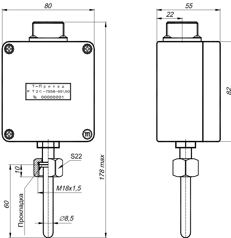
Малюнок 1 – Габаритні розміри РТ2С-7558.
