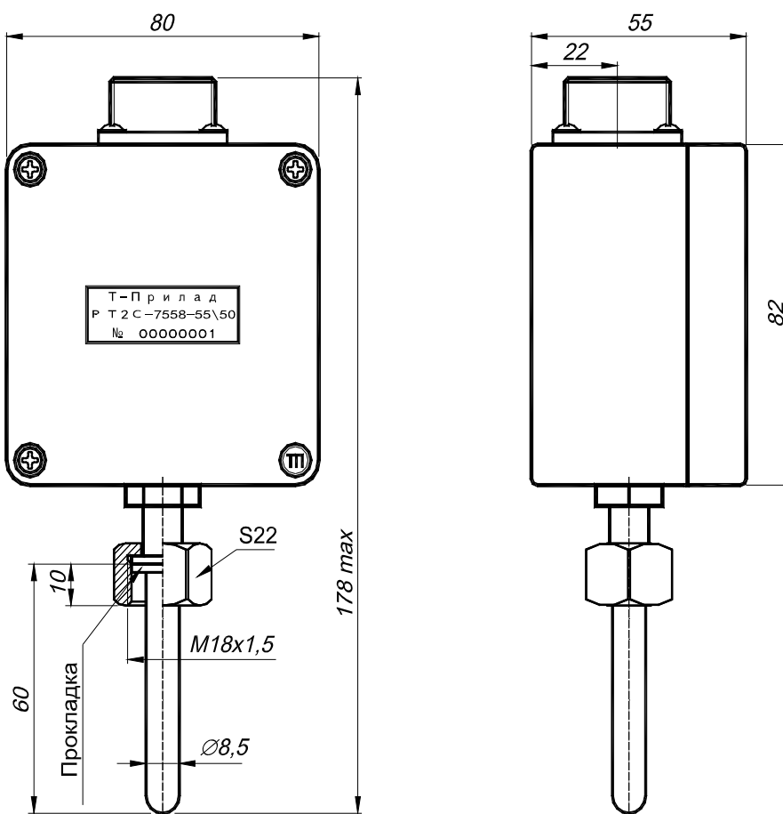
Рисунок 1 – Габаритные размеры PT2C-7558.
